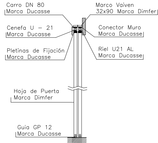
Caso A - Sistema Fuera de Vano
