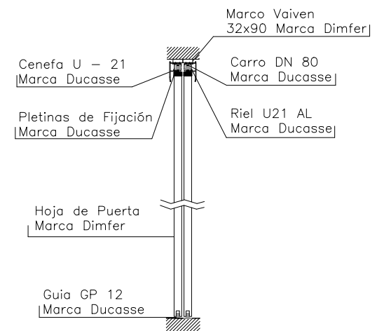
Caso B - Sistema Dentro de Vano
